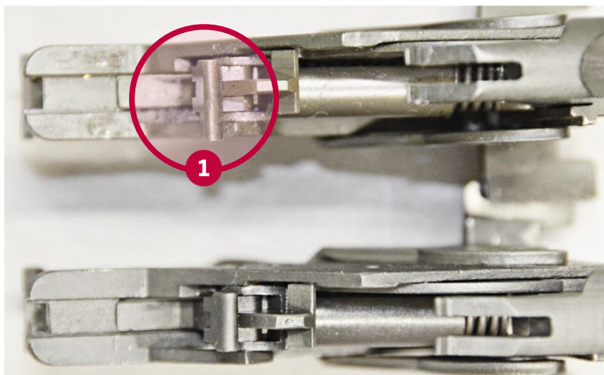
Abbildung 60 Untere Gehäuseteile M 14 und M 1A, oben gut erkennbar der Dauerfeuerhebel des Springfield M 14
